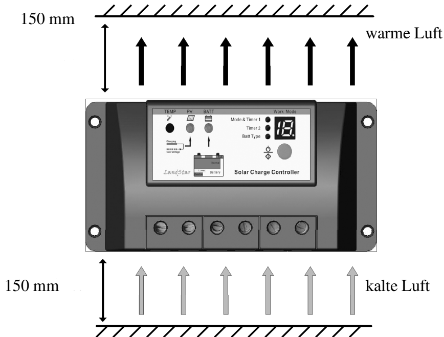
Bild 3-1 Montage und Kühlung
