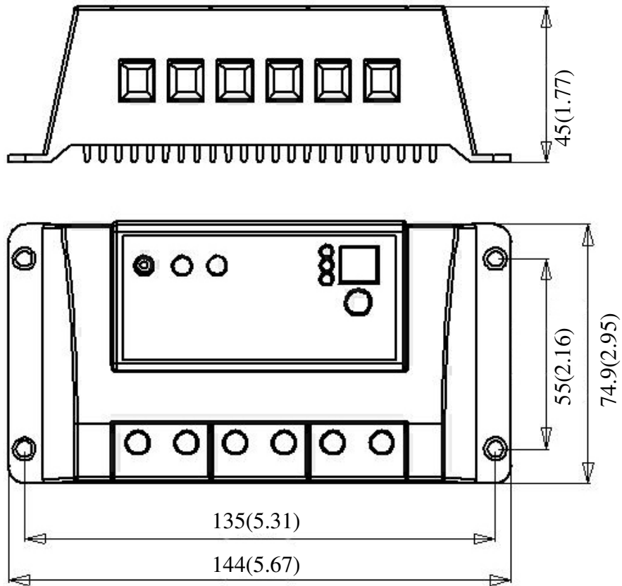
Bild1-2 LS1524R & LS2024R Dimensionen
