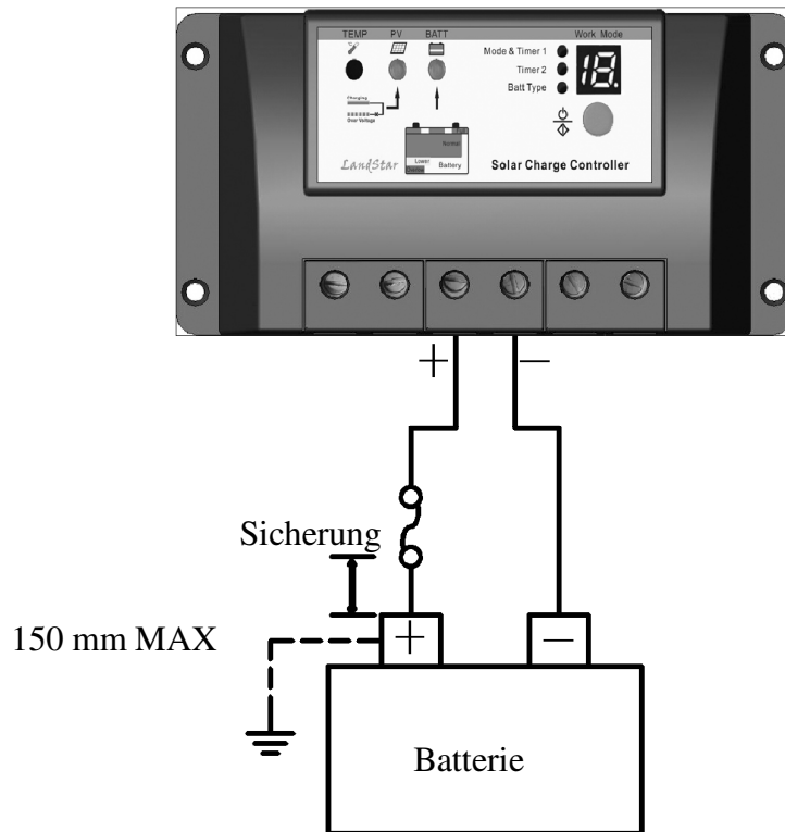
Bild 3-2 Batterieanschluss
