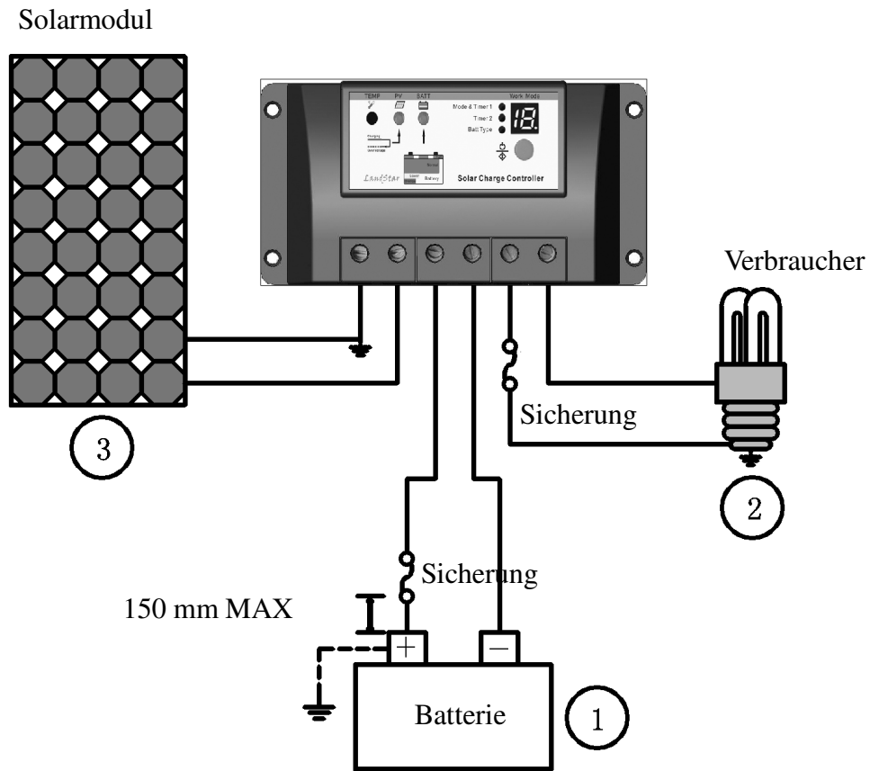
Bild 3-5 Systemanschluss
