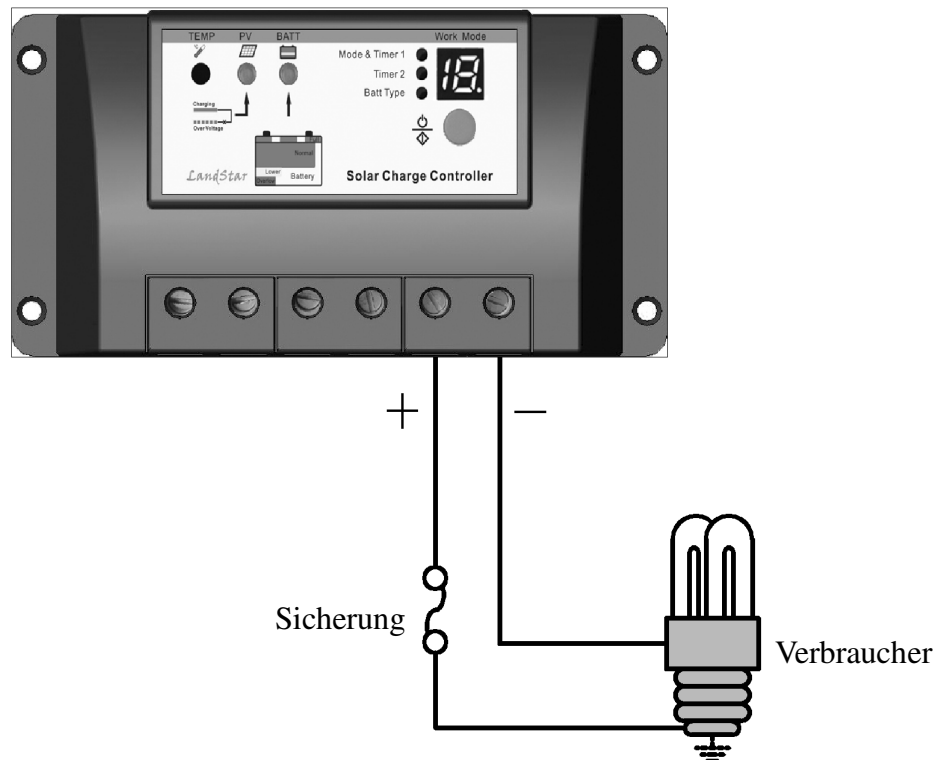
Bild 3-3 Verbraucheranschluss
