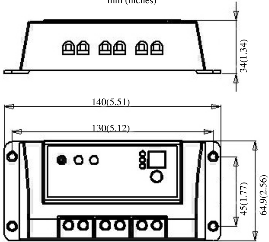
Bild1-1 LS1024R Dimensionen
